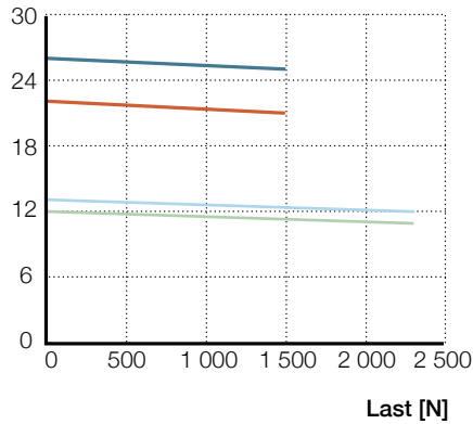
Geschwindigkeit/Last Diagramm
