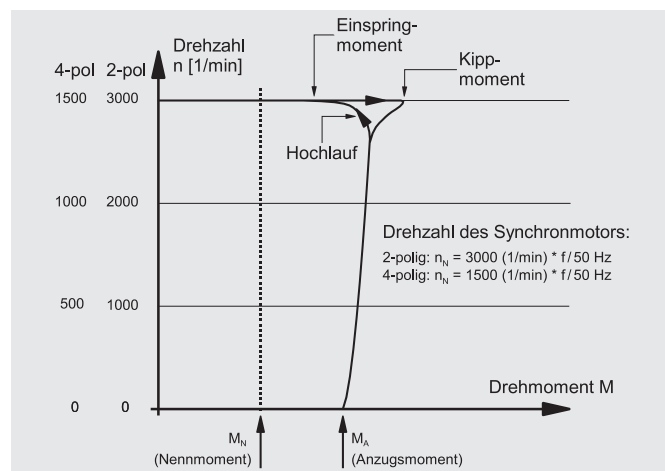
Zusammenhang von Drehzahl und Drehmoment beim Synchronmotor
