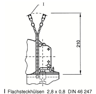
Anschluss K191
