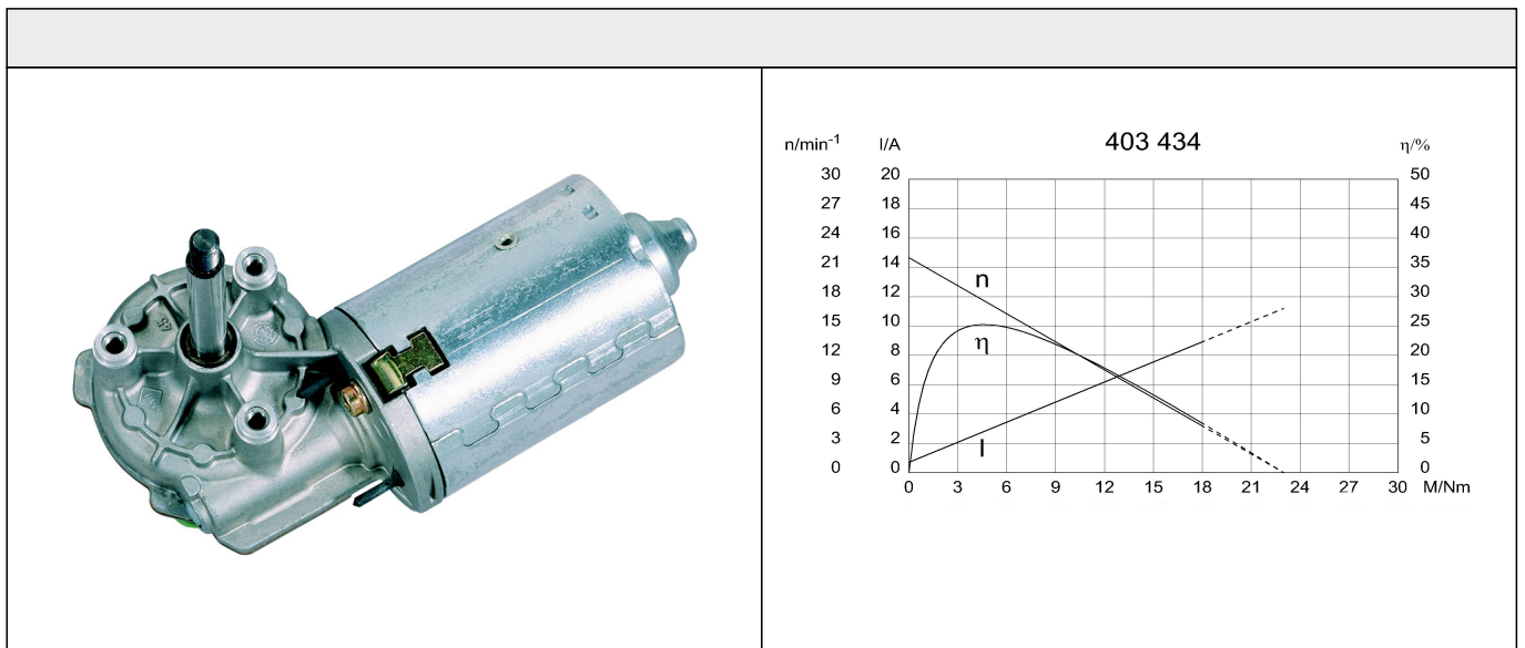
Abtriebswelle W120
