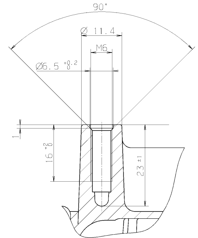
Schnittansicht der Befestigungsdome
