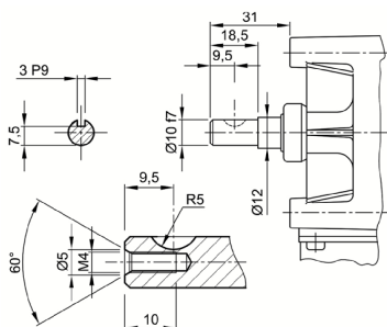
Abtriebswelle W191
