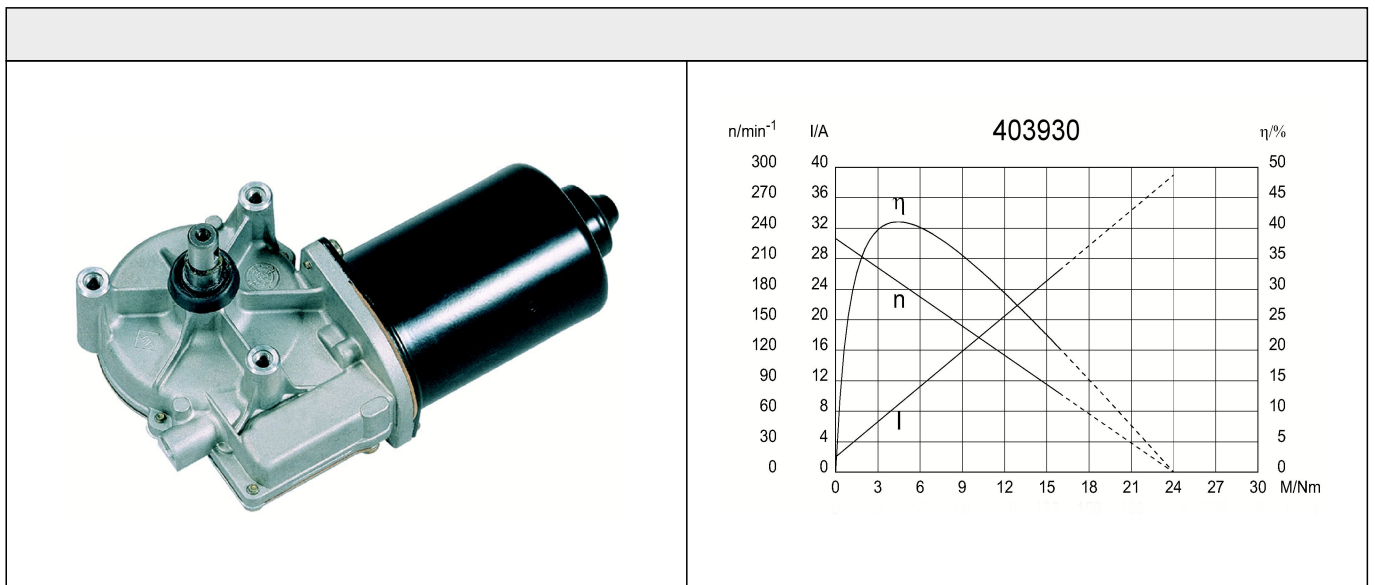
Abtriebswelle W191
