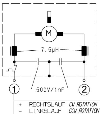
Schaltbild S404157
