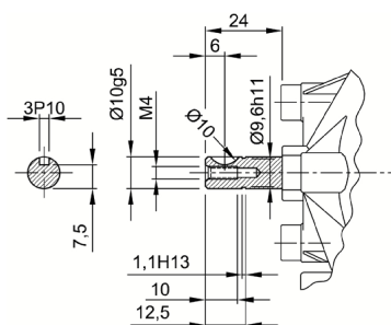
Abtriebswelle W304
