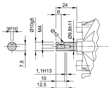
Abtriebswelle W304
