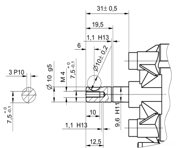
Abtriebswelle W328
