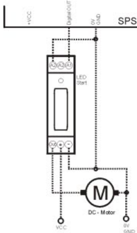
SPS - Beschaltung
