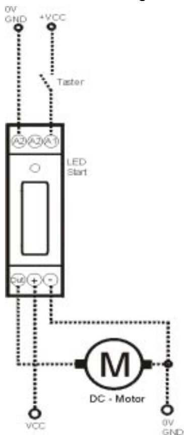
Standard - Beschaltung
